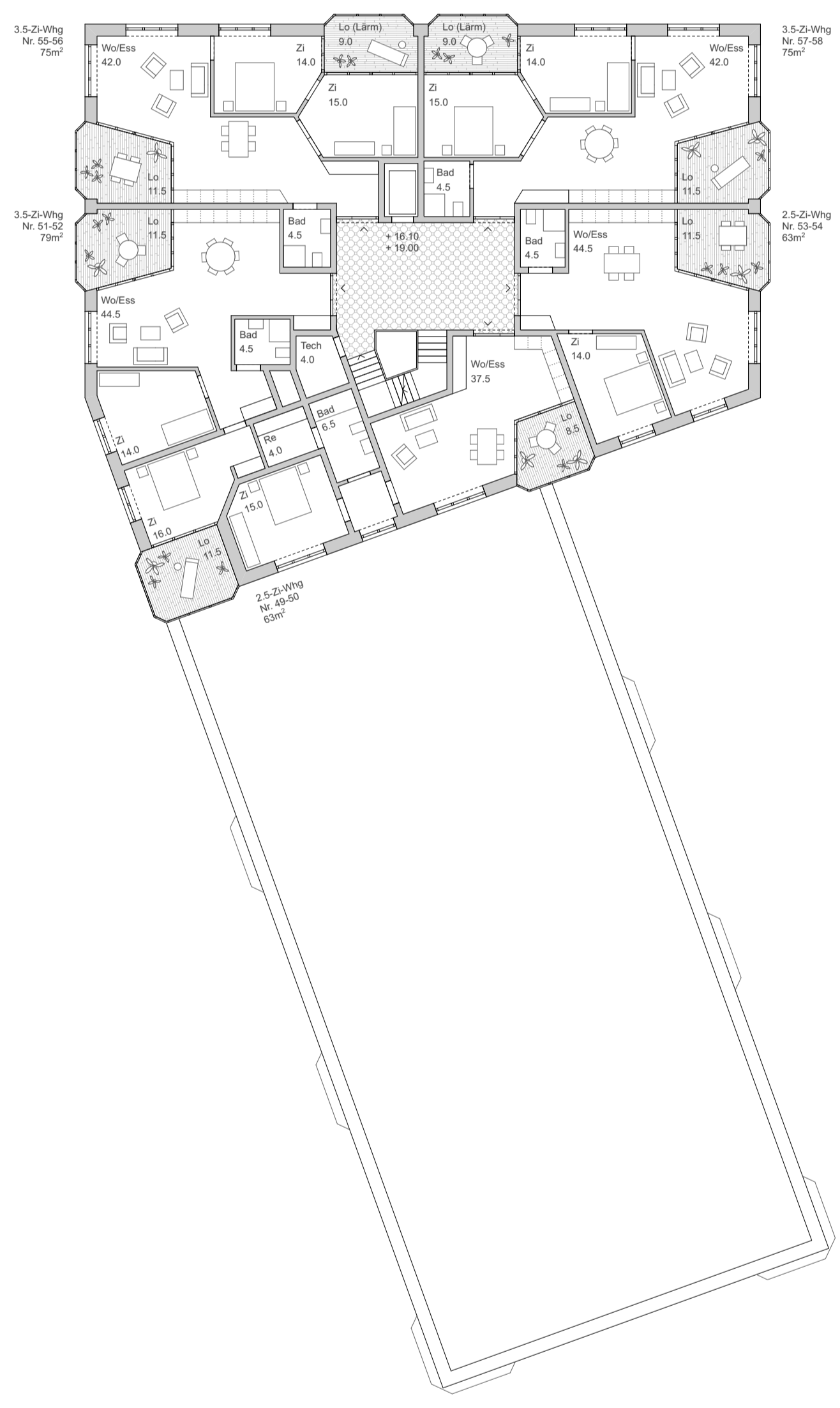
5./6. Obergeschoss 1/200
